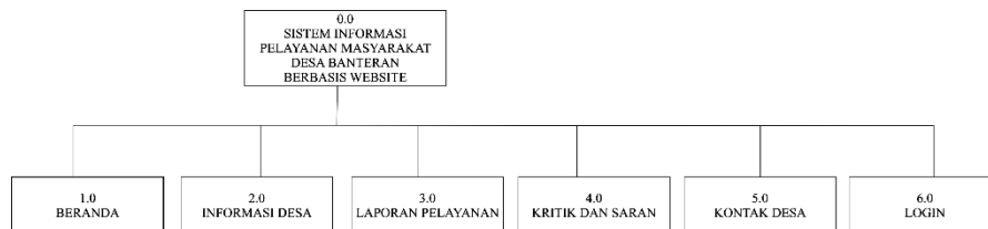
Gambar 1. VTOC UserUmum
